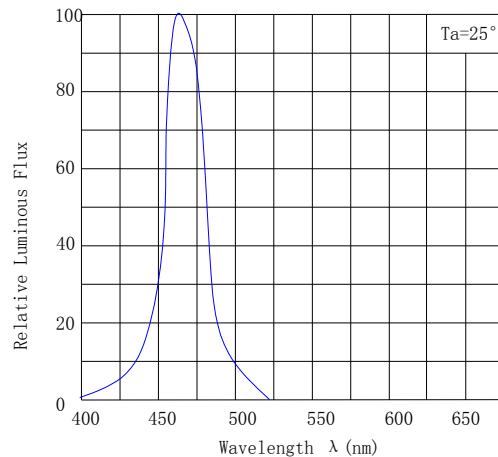
Wavelength Characteristics 相对光谱分布曲线图
